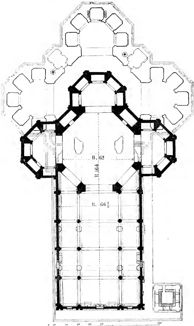
Scala di Grazia Fiorentina: Grundriß des Doms von Florenz.
